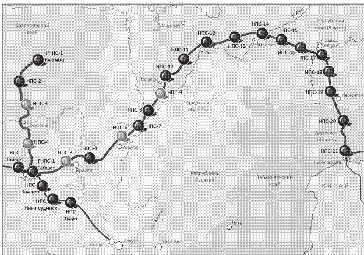
Рис. 1. Трасса трубопровода «Восточная Сибирь – Тихий океан»
